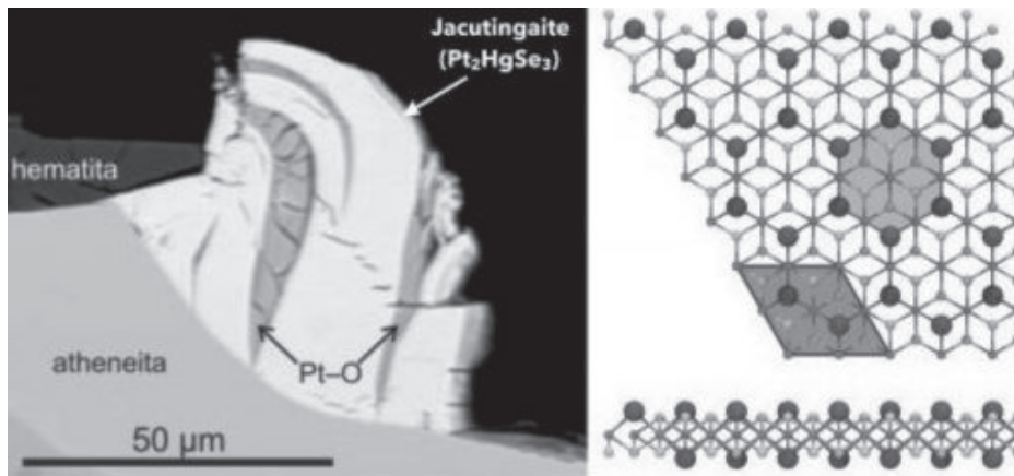
Imagem por microscopia eletrônica da jacutingaíta (branco) sobre a superfície de um bloco de hematita, potarita e ateneita. À direita, visão superior e lateral de uma camada monoatômica de jacutingaíta
